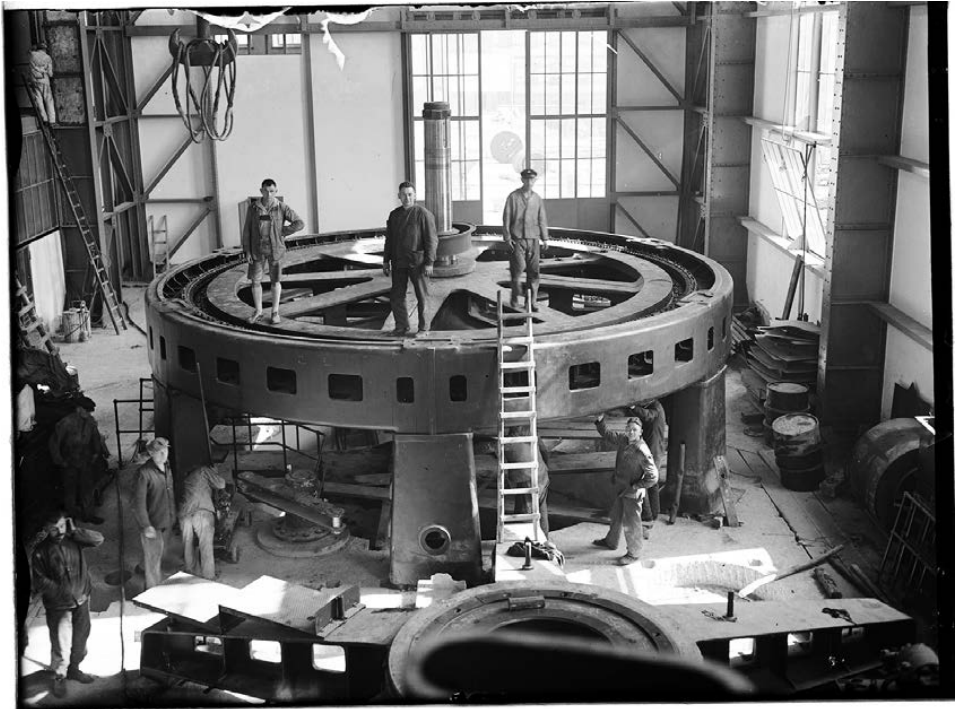
Bau der Staustufe Klingenberg 1930
